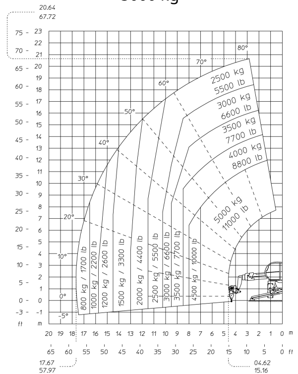
Rotation sur stabilisateurs abaissés avec treuil 5000 kg
