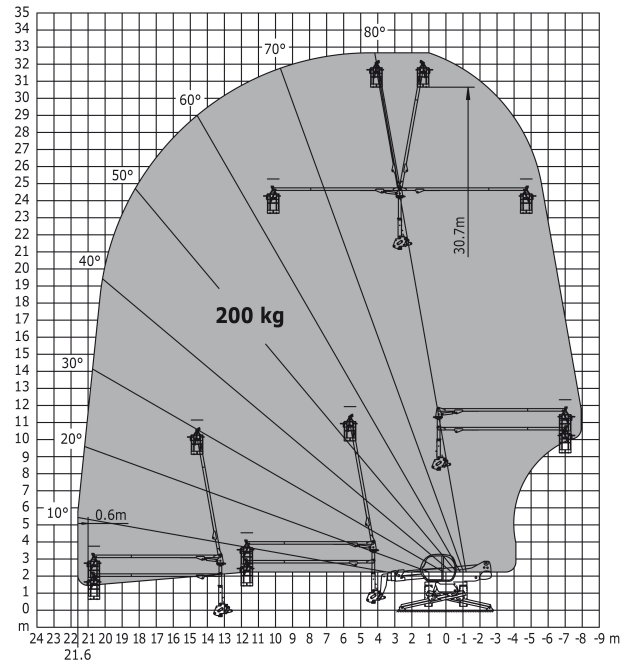
Rotation sur stabilisateurs abaissés avec 3D positif
