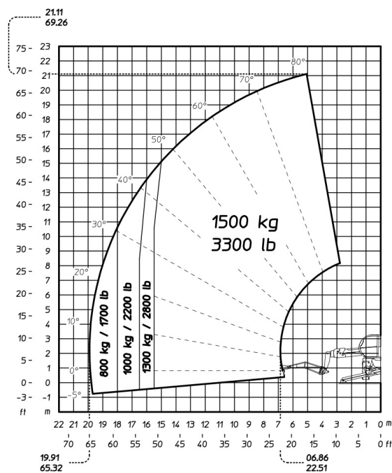
Rotation sur stabilisateurs abaissés avec potence 1500 kg
