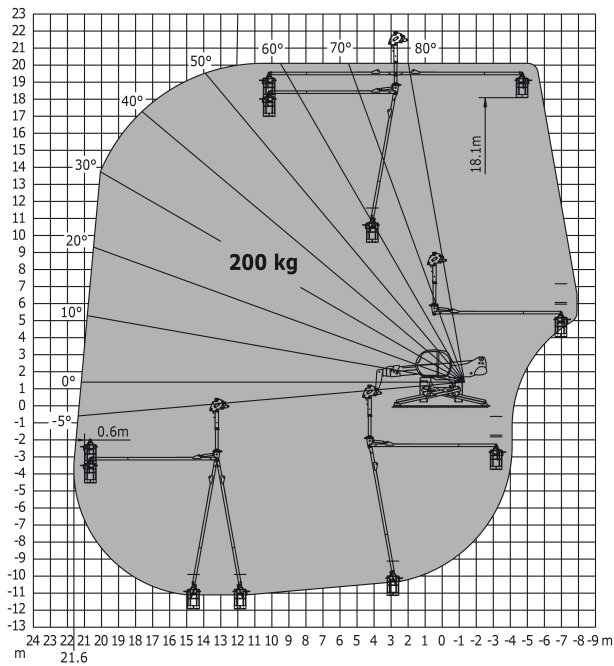
Rotation sur stabilisateurs abaissés avec nacelle 3D négatif
