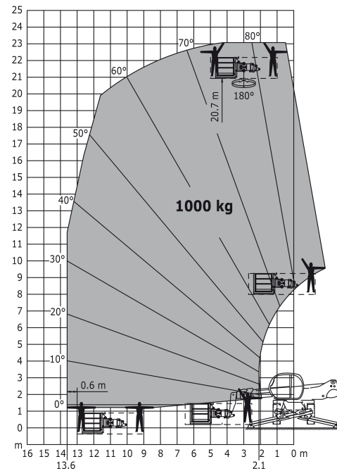
Rotation sur stabilisateurs abaissés avec nacelle 1000 kg
